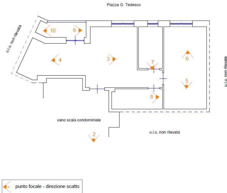
Pianta piano ottavo Stato dei luoghi
