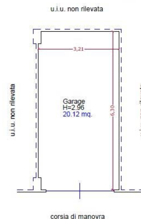
Pianta piano seminterrato Stato dei luoghi
