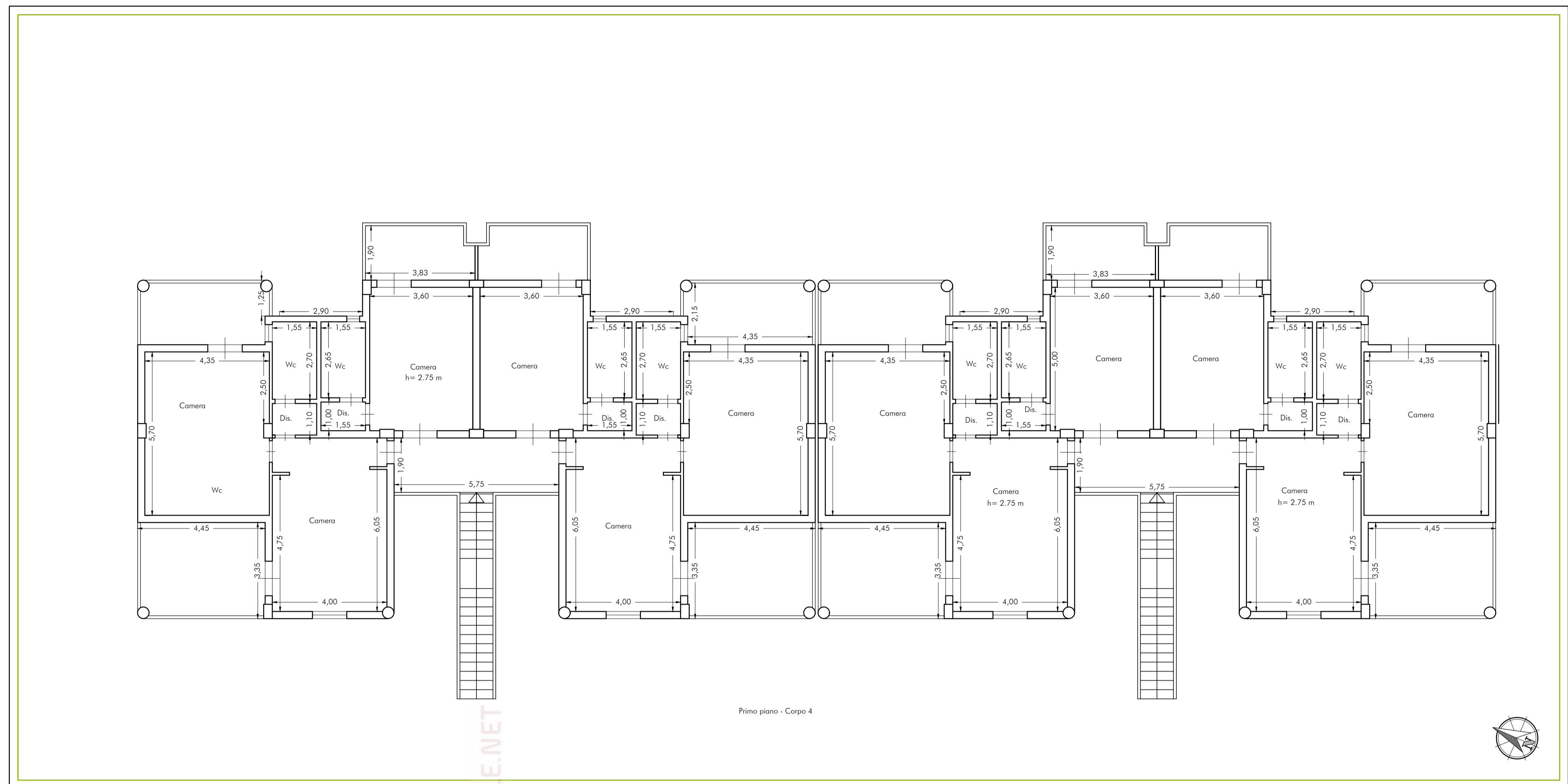
Planimetria piano primo - CORPO 4 - Scala 1:100
