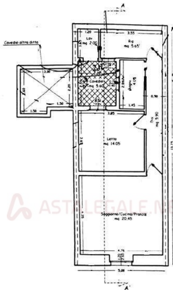
PIANTA PIANO TERRA Stato di progetto
